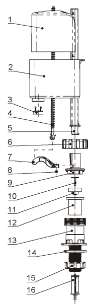
Рис. 1 - Клапан впуска (нижняя подводка)
