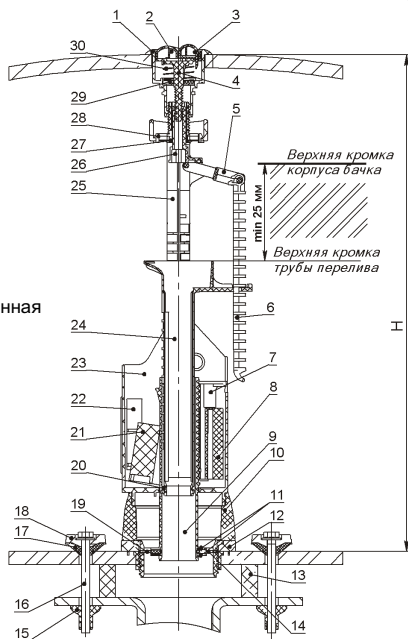
Рис. 2 - Клапан выпуска
